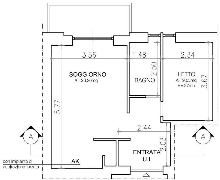
STATO ATTUALE SCALA 1:100
