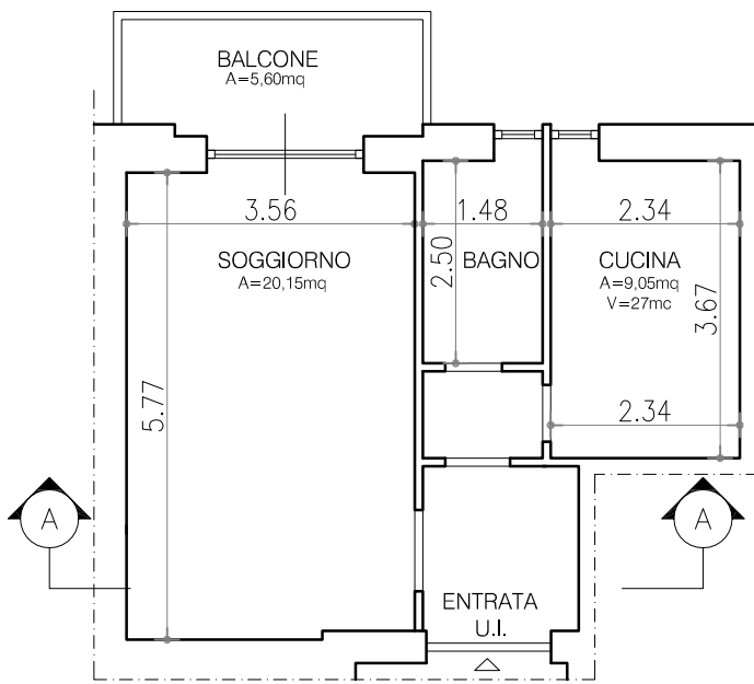
STATO Licenza Edilizia 299/1955 prot. 39710 SCALA 1:100
